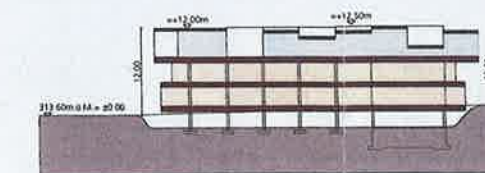
Querschnitt C-C
