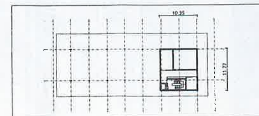
2. Untergeschoss: Keller
