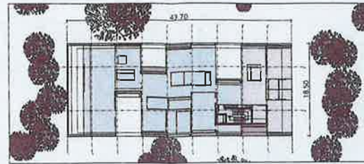
Dachgeschoss: Wohnung
