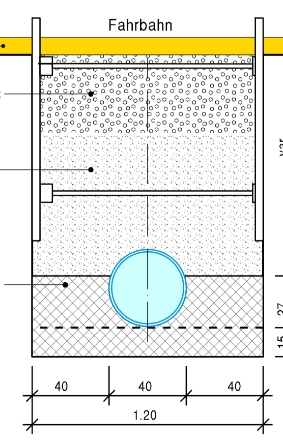
Grabenprofil 1:20 PROJ. RAW-KANAL PE 400/375
