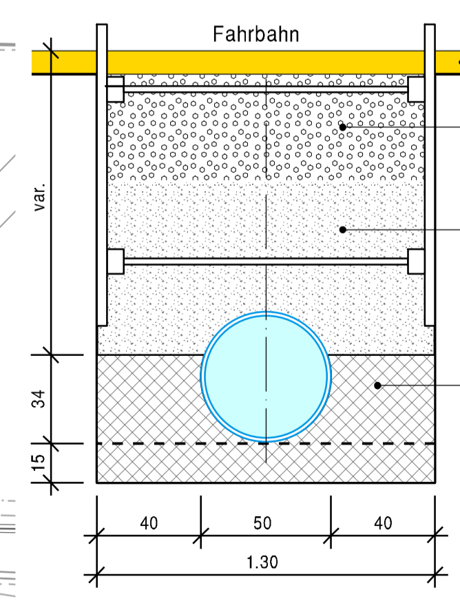
Grabenprofil 1:20 PROJ. RAW-KANAL PE 500/469
